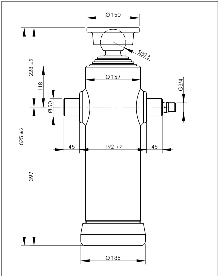
Scala - Scale - Échelle - Maßstab: 1:5
