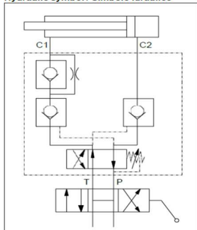
Hydraulic symbol / Simbolo idraulico
